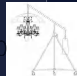
1111F L3800×W1800×H(2880~3210)
