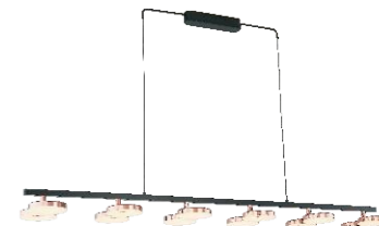
# 6165S-L12-LED ☏ Pendant Lamp Ⓢ 26*147*180cm 💡 LED 12*6W Ⓜ aluminium/PE Ⓢ 黑+玫瑰金
