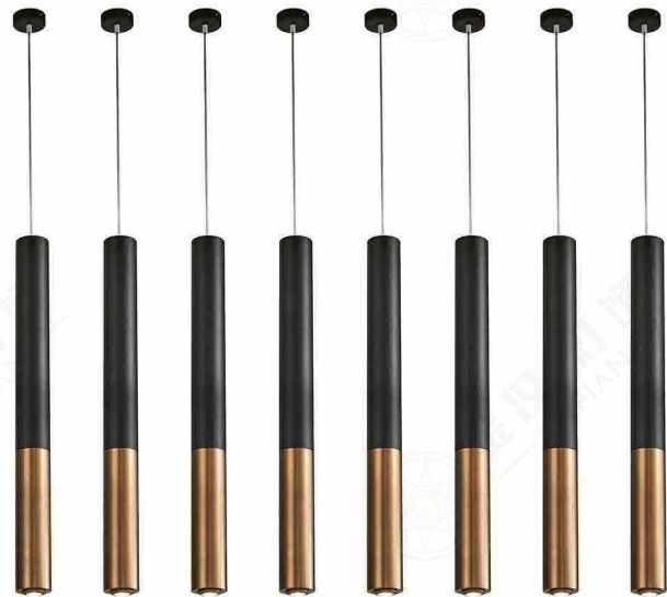
JH51326-1 (单个) 尺寸Size: D76*H1500mm 光源Bulb: GU10 颜色Colour: 哑黑色漆+拉丝青古铜 材质Material: 不锈钢
