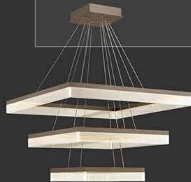
MA05632P-003 (800*800+600*600+400*400) power : LED 141W 3000K size : 8900 W800 H1500mm colour : coffee material : aluminum+Acrylic
