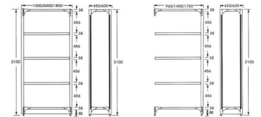
OW-T01A 基础架
