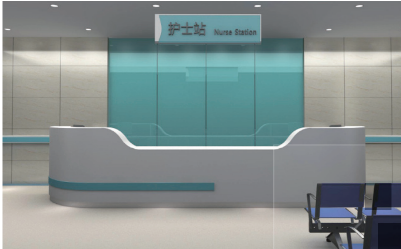
U型护士站 NS01-UXXX75-MB 规格:W5200xD750/W2000xD750/H1150
